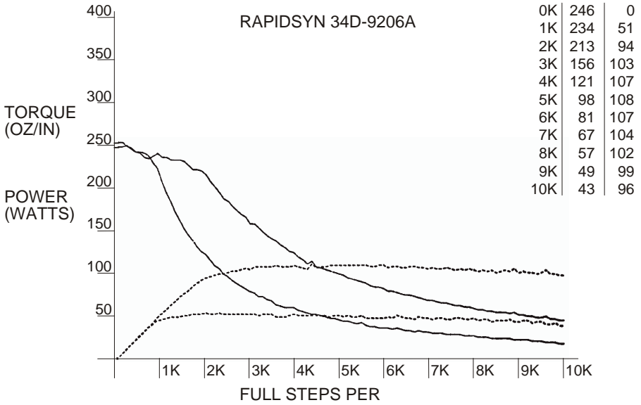
Figure 23 - RAPIDSYN 34D-9206A
