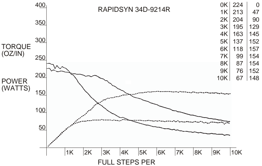
Figure 16 - RAPIDSYN 34D-9214R
